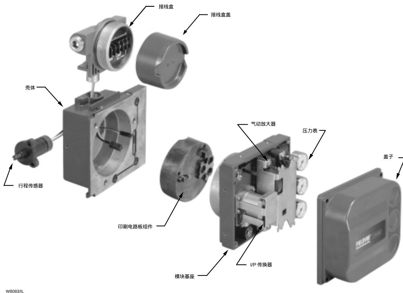
图 9. DVC6000 系列数字式阀门控制器组件
