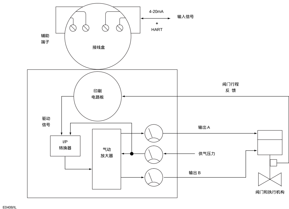
图 10. DVC6000 系列数字式阀门控制器方块图
