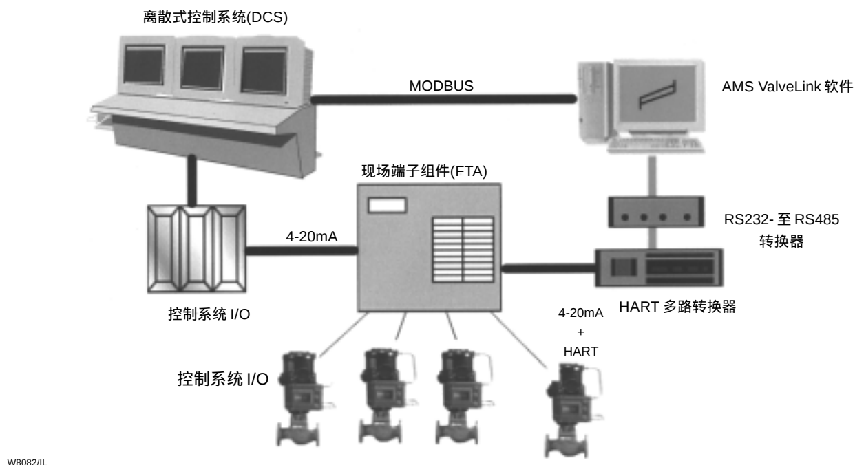
图 5. 通过 AMS ValveLink 软件的 Modbus 界面将来自数字式阀门控制器的信息集成到非 HART 兼容的控制系统中去
